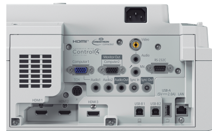
Porta USB-A adicional na lateral do projetor.
