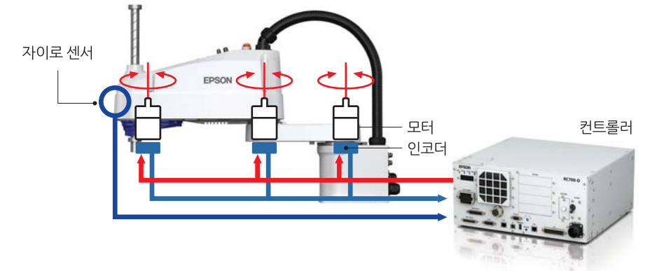
진동이 억제되지 않는 로봇
